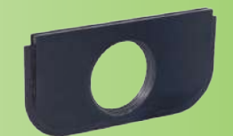
Un perçage taraudé 1"BSPP pour pied de traçage ou presse étoupe
